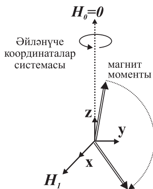
1 нче рәсем. ЭПР күренешенә классик интерпретациясе.
