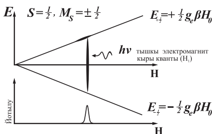
2 нче рәсем. ЭПР күренешенә квант-механик интерпретациясе.
