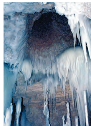
Юрбев мәгарәсе. Боз сталактитлары булган карст коесы.
