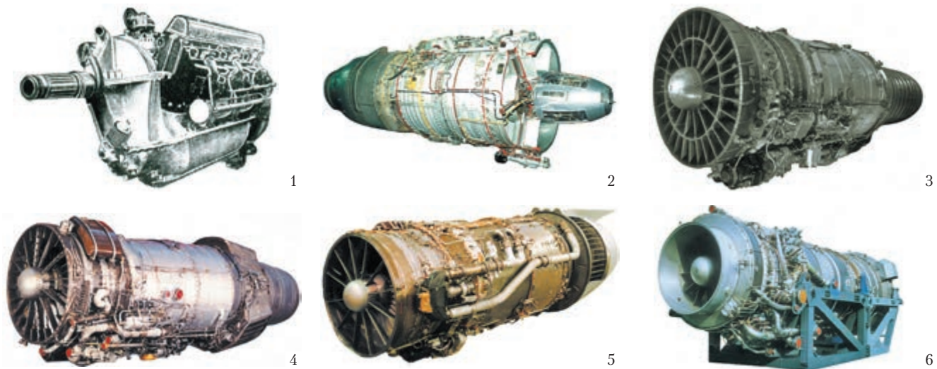
Авиация двигательләре. 1. ВК-105ПФ; 2. РД-3М-500; 3. НК-8-4; 4. НК-8-2У; 5. НК-86; 6. НК-16-18СТ.
