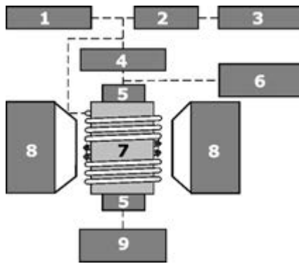
Акустик парамагнетик спектротметрның блок-схемасы.
