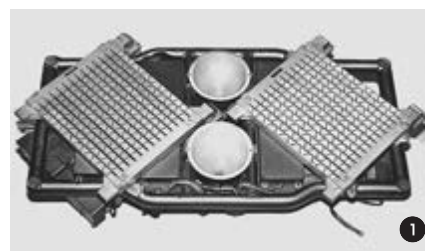
Антенна системалары: 1) рупорлы һәм ярыклы 2) рәшәткәле; 2) киң полосалы 2 вибраторлы.
