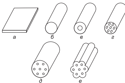
Дары корылмалары (зарядлары) элементлары: а) пластина, б–е) бөртек һәм бер яки берничә каналлы көпшә.
