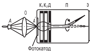
Электрон-оптик әверелдергеч.
