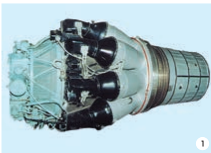
Двигательләр төзү. 1. МиГ-15 самолеты өчен В.Я. Климов конструкциясе буенча эшлэнгән ВК-1 двигателе; 2. Газ суырту агрегатлары (ГПА) өчен НК-38СТ двигателе; 3. «КАМАЗ-65115-04» автомобиленең егрәлек агрегаты.
