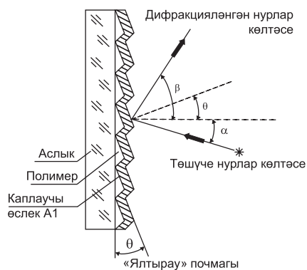
1 рәсем. Кайтаручы дифракцион рәшәткә.
