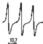
Эремәдәге (T=293K) нитроксиль И.р. ЭПР спектрының үтә нәзек структурасы.
