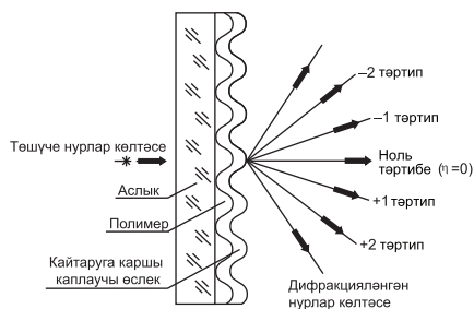
2 рәсем. Үткәрүче дифракцион рәшәткә.
