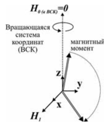
Рис. 1. Классическая интерпретация явления ЭПР.
