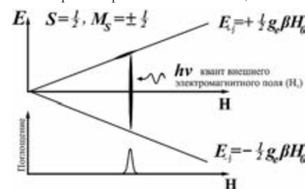
Рис. 2. Квантово-механическая интерпретация явления ЭПР.
