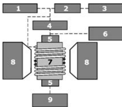
Блок-схема акустического парамагнитного спектрометра.
