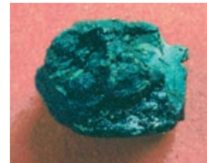
Асфальтит из Шугуровского месторождения битумов.
