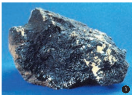
1. Битум с Шугуровского месторождения; 2. Битуминозный песчаник из нижнеказанских отложений.
