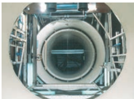
Испытание модели моста в аэродинамической трубе Т-1К.
