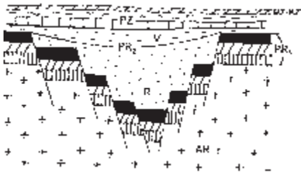
Схематический разрез авлакогена Восточно-Европейской платформы.
