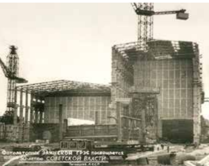
Идел буендагы иң зур дәүләт район электр станциясе төзелеш. Зәй ГРЭСы. 1960 еллар
